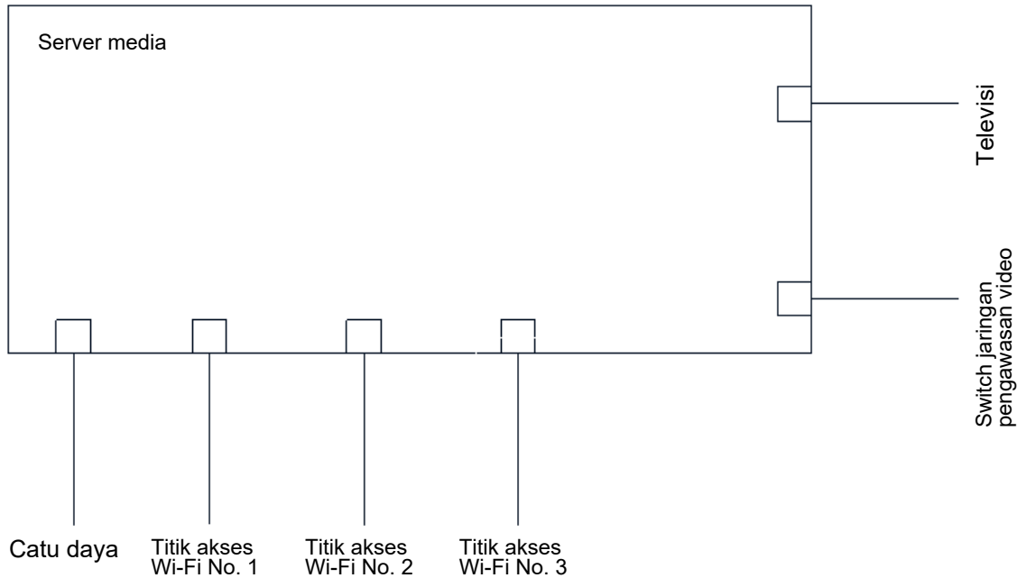
Diagram koneksi
