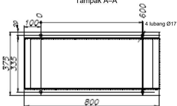
Tampak A-A
